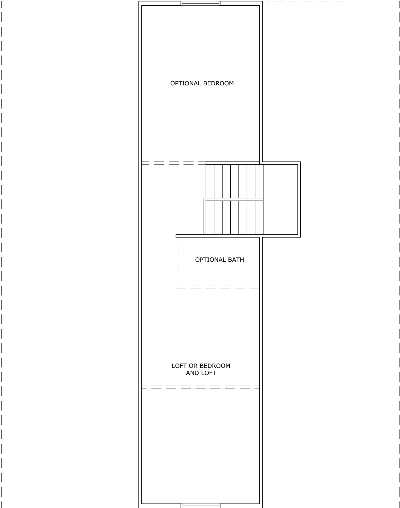
OPTIONAL LOFT PLAN 696 S.F.
